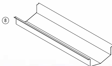
21x200 0003630 CANALETTA INOX CON FORO E FLANGE DI TESTA STAINLESS STEEL GUTTER WITH HOLE AND END FLANGES
